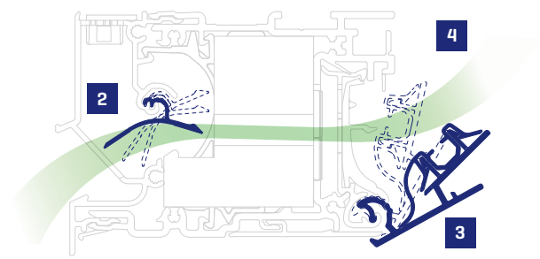
Invisivent® COMFORT
